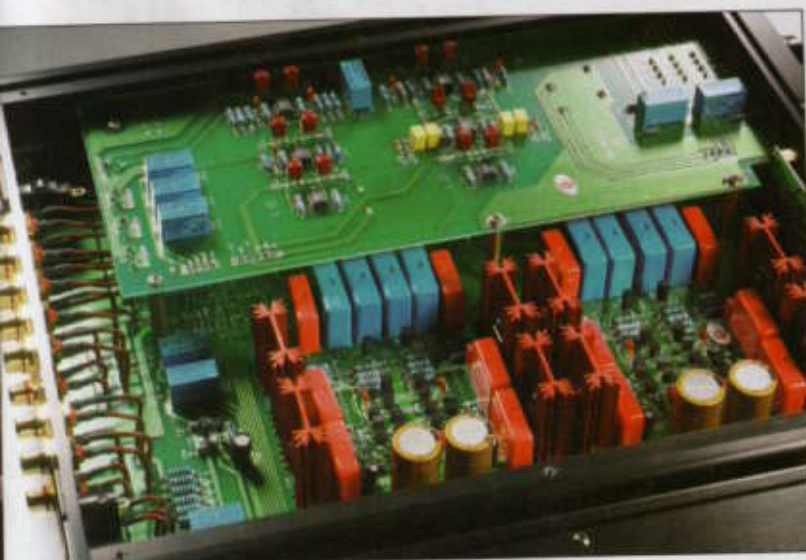
Der Preamp glänzt mit einem vorbildlichen Platinen-Layout. Die Kanäle sind strikt voneinander getrennt. Recht kräftige Kabel führen die Signale von den Ein- und Ausgangsbuchsen zu den Verstärkerstufen.
