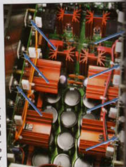
Die Leistungshalbleiter (Pfeile) sitzen direkt an den massiven Aluprofilen rechts und links. Schon im Leerlauf erwärmen sie das Gehäuse der Endstufe kräftig.
